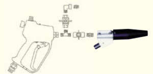
Handtag med fjärrstyrning av lufttryck, start/stopp samt reglage av vattenflöde.
